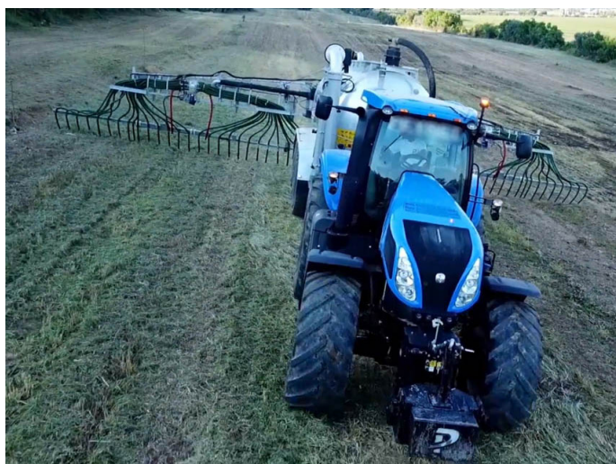
Aplicador de purín Vogelsang Swin Up 2 Farmer 30+30 salidas
